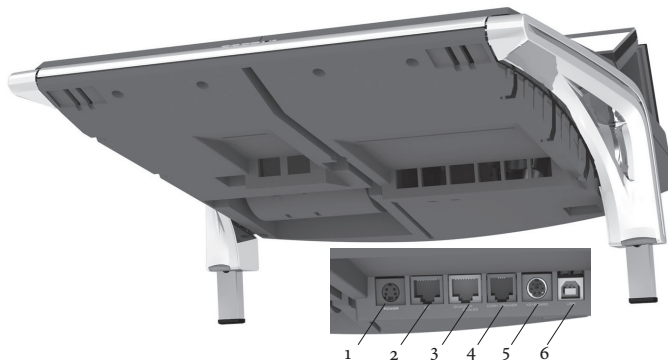
< Obrázok 2.3 Zadní konektory pokladny Euro-2100.
